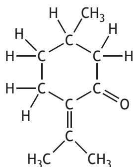
pulegone
